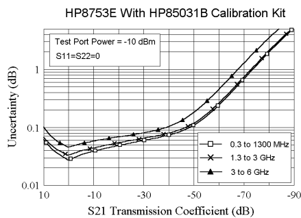
Magnitude
