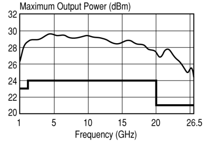
83018A Amplifier
