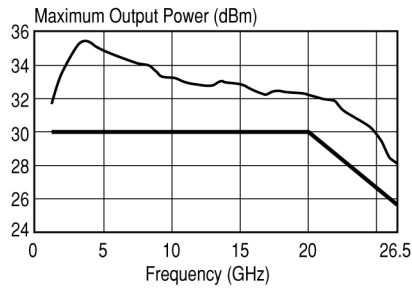
83020A Amplifier
