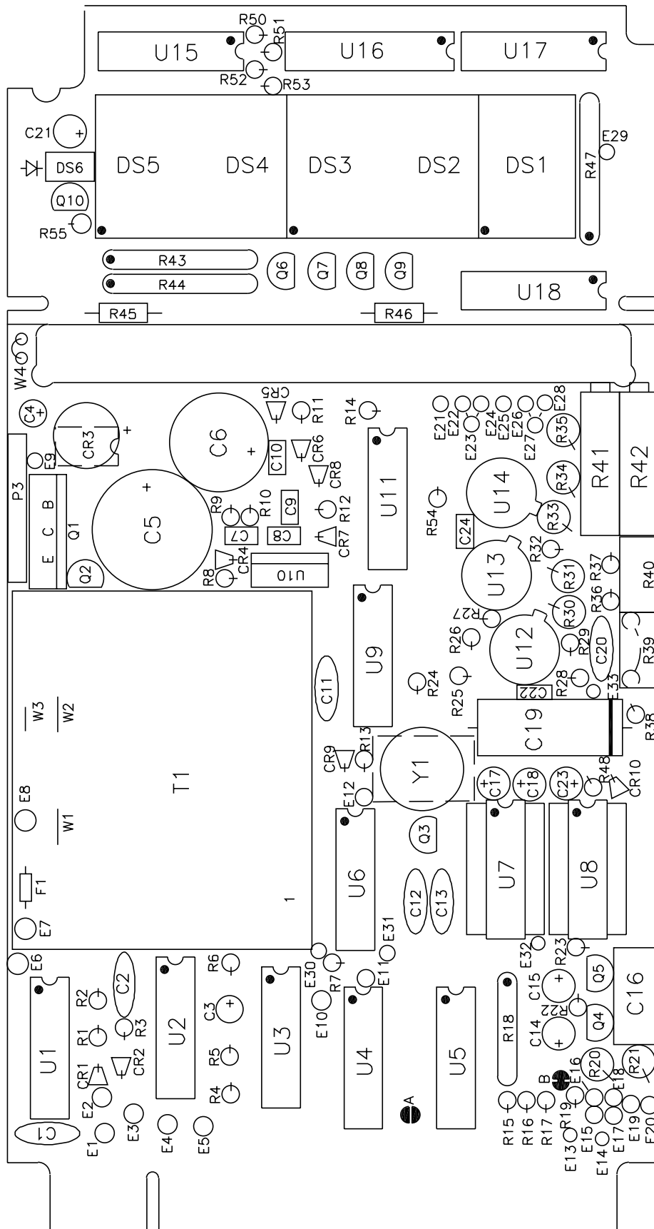
PCBA DWG, 2003B, 4 1/2 DIGIT DPVM
